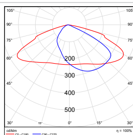
Curva Luminotécnica 100W
