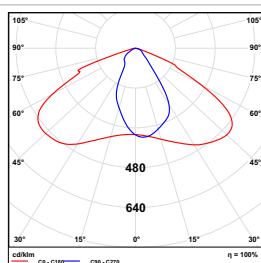
Curva Luminotécnica 50W
