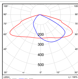
Curva Luminotécnica 120W
