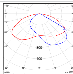
Curva Luminotécnica 180W
