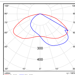
Curva Luminotécnica 150W
