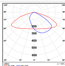
Curva Luminotécnica 80W
