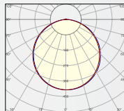
Curva IES de referência • 200.74.0220
